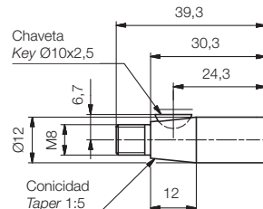
Eje forma Z / Shaft form Z
