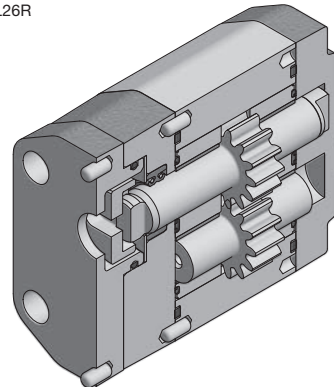
Bomba trasera con eje tipo L y tapa tipo 26 Rear pump with shaft form L and front flange type 26
